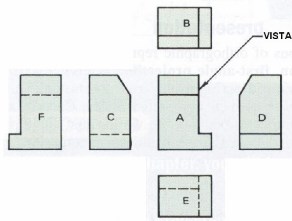
(C) COLOCACIÓN DE LAS VISTAS EN LA SUPERFICIE DE DIBUJO
