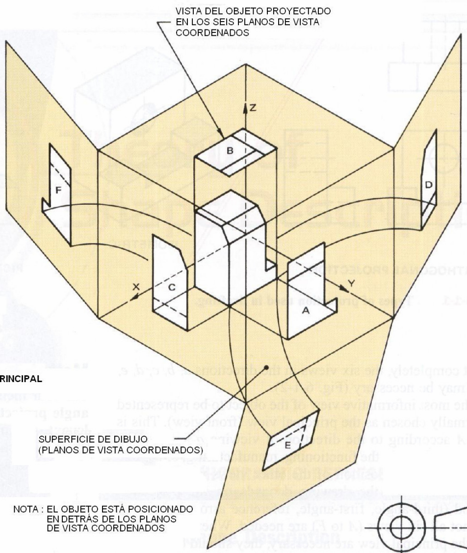
(B) DISPOSICIÓN DE LA SUPERFICIE DE DIBUJO
