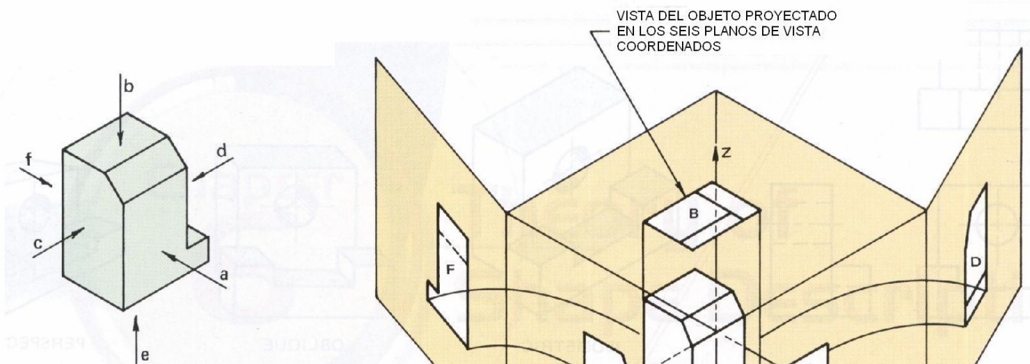
(A) DIRECCIONES DE LAS VISTAS
